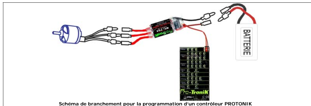
Schéma de branchement pour la programmation d'un contrôleur PROTRONIK
